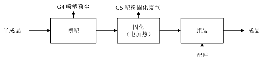
图2-3 喷塑线生产工艺流程及产污环节示意图
