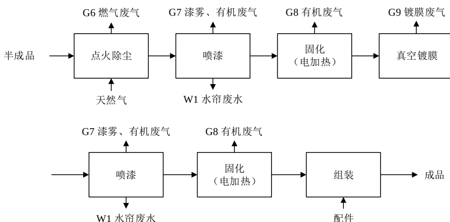
图2-4 喷漆线生产工艺流程及产污环节示意图
