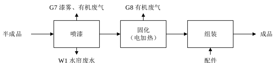
图2-5 手工喷漆生产工艺流程及产污环节示意图
